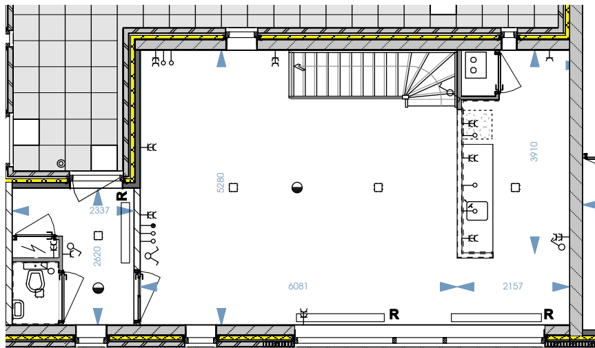
1e verdieping
