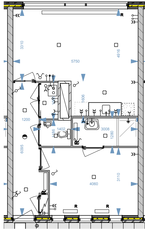
type C1 bouwnummer 5 t/m 7 + 20 t/m 22
